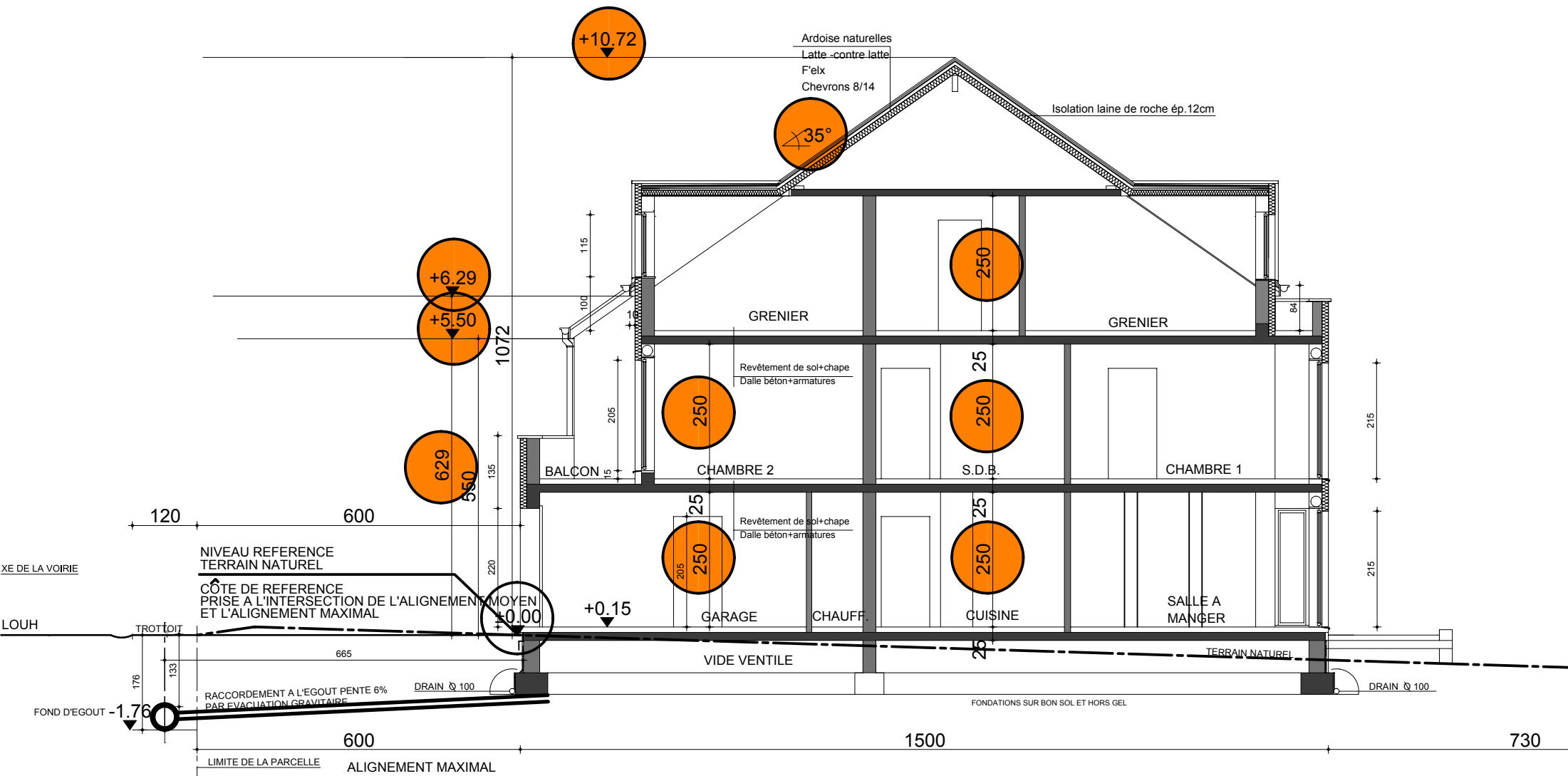
COUPE A- B
